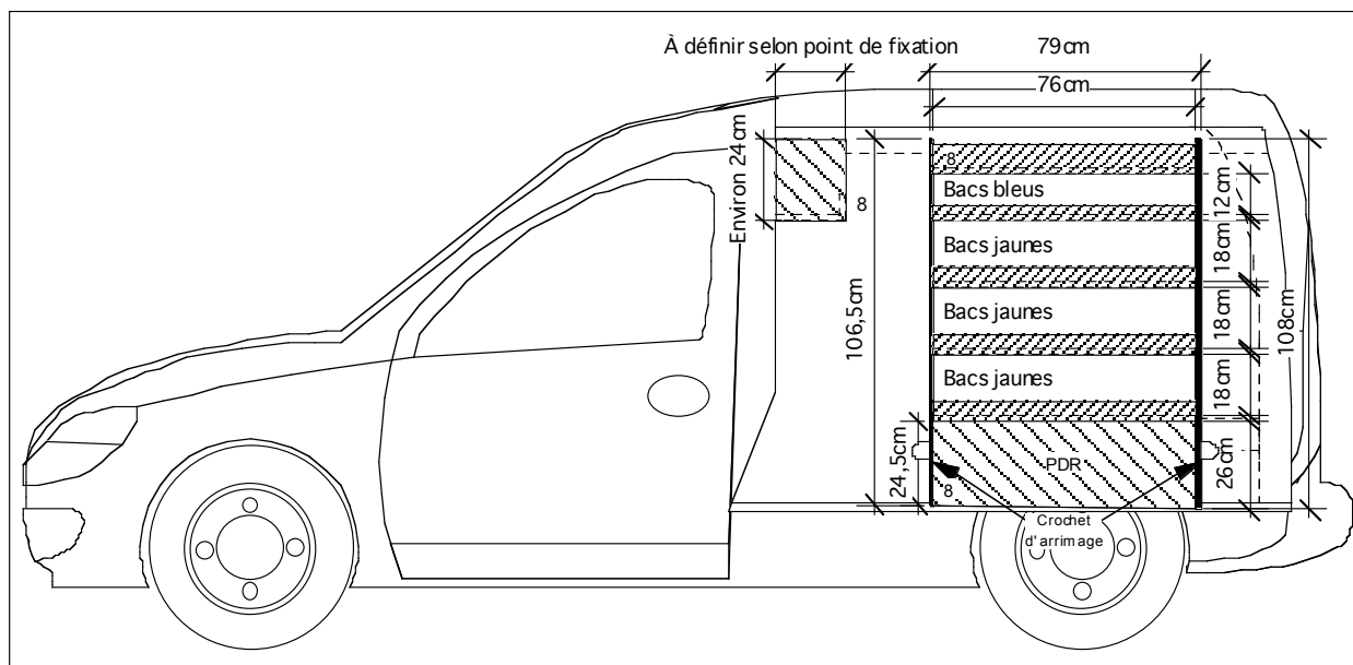
AGENCEMENT COMBO PL Vue en coupe de l'aménagement intérieur : côté droit
