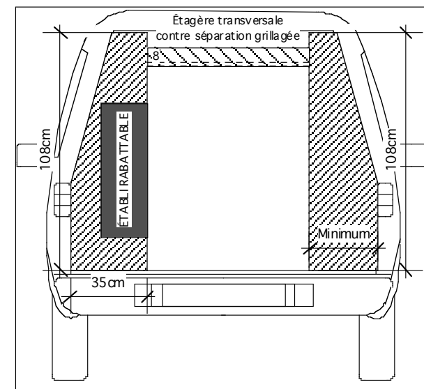
AGENCEMENT COMBO PL Vue en coupe de l'aménagement intérieur : côté arrière
