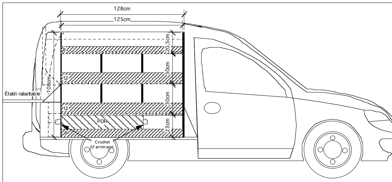
AGENCEMENT COMBO PL Vue en coupe de l'aménagement intérieur : côté gauche
