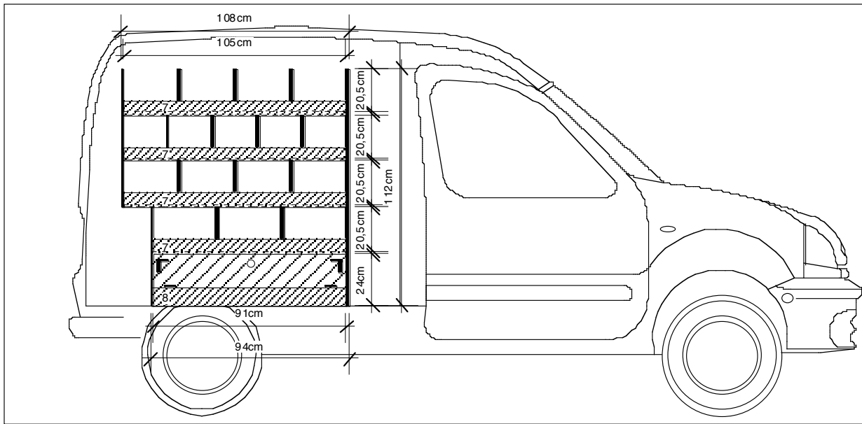
AGENCEMENT KANGOO PL VUE GAUCHE
