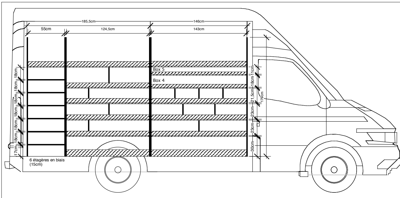
AGENCEMENT IVECO L3 VUE GAUCHE
