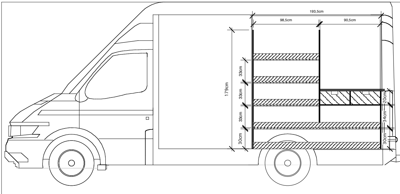
AGENCEMENT IVECO L3 VUE DROITE
