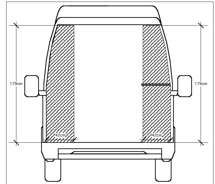
AGENCEMENT IVECO L3 VUE ARRIERE
