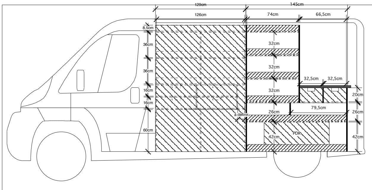
AGENCEMENT DUCATO L2H2 Vue en coupe de l'aménagement intérieur : côté droit
