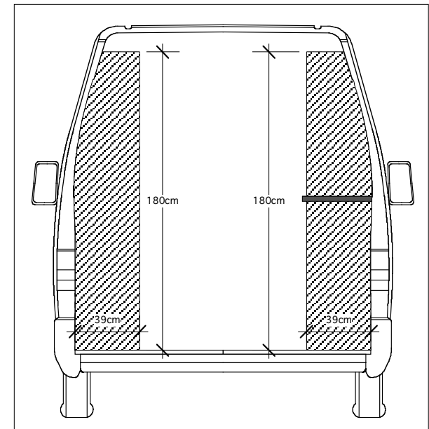
AGENCEMENT DUCATO L2H2 Vue en coupe de l'aménagement intérieur : côté arrière
