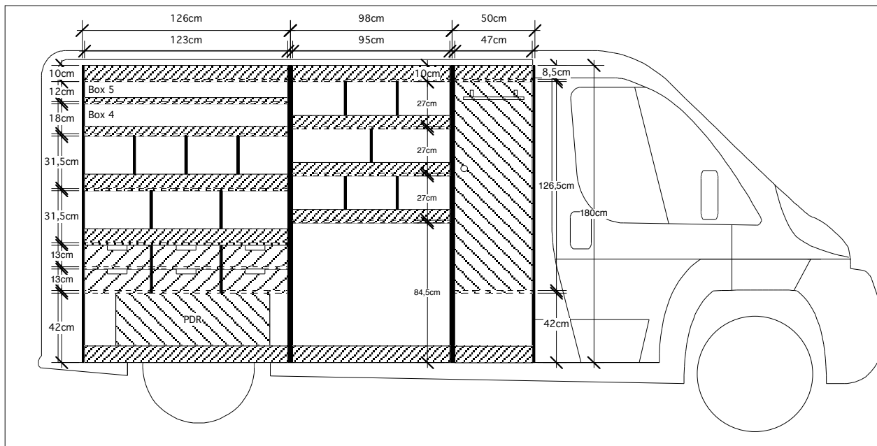
AGENCEMENT DUCATO L2H2 Vue en coupe de l'aménagement intérieur : côté gauche
