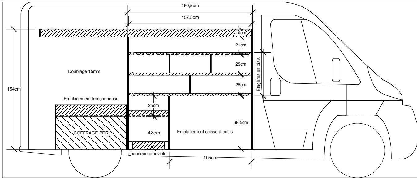
AGENCEMENT DUCATO L2H1 Vue en coupe de l'aménagement intérieur : côté gauche
