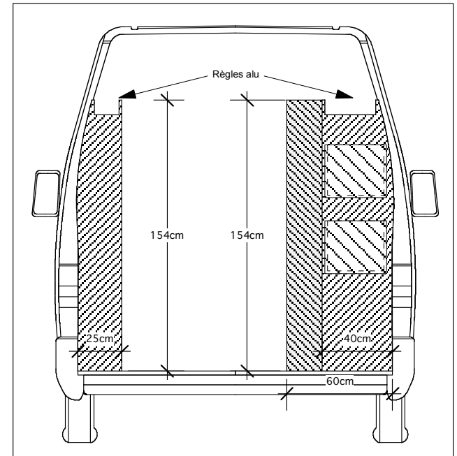
AGENCEMENT DUCATO L2H1 Vue en coupe de l'aménagement intérieur : côté arrière
