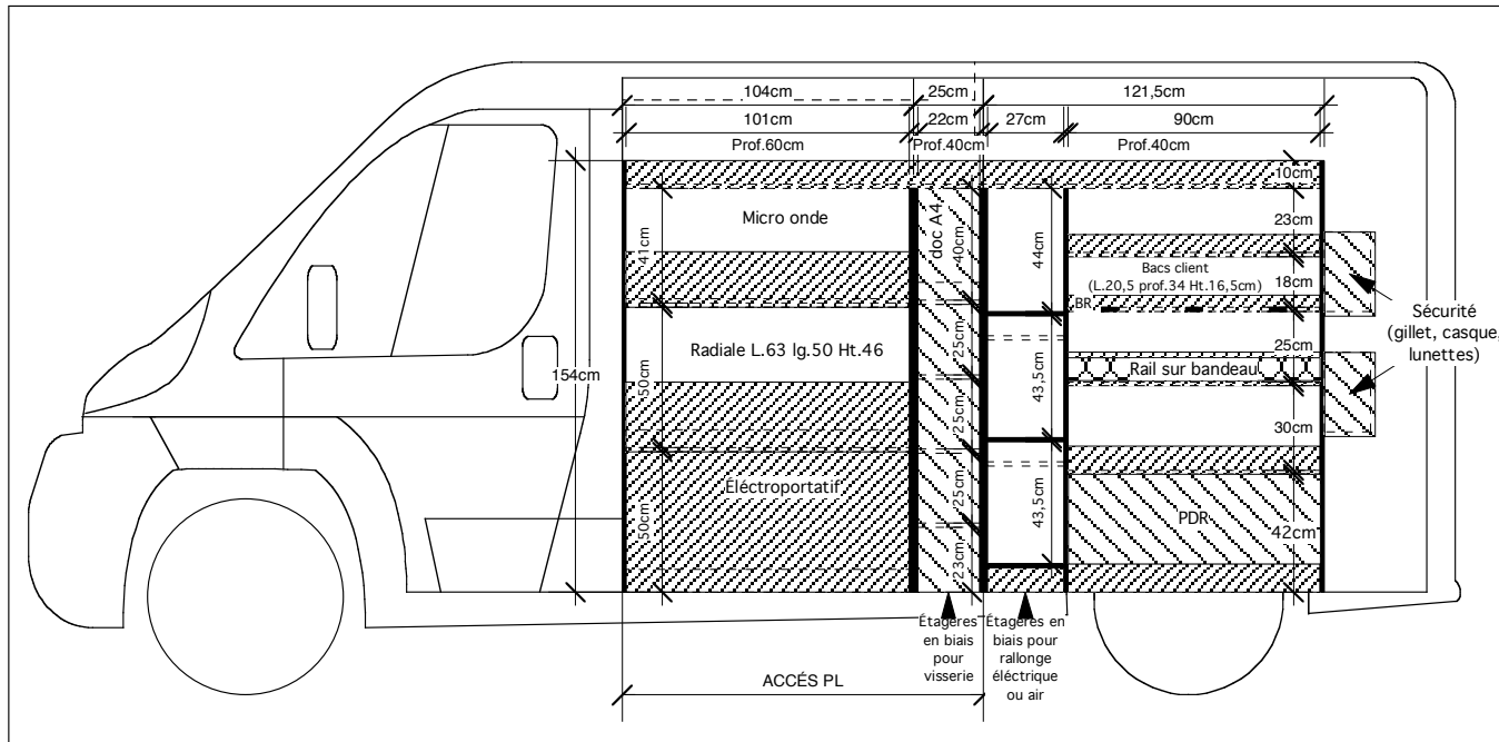
AGENCEMENT DUCATO L2H1 Vue en coupe de l'aménagement intérieur : côté droit
